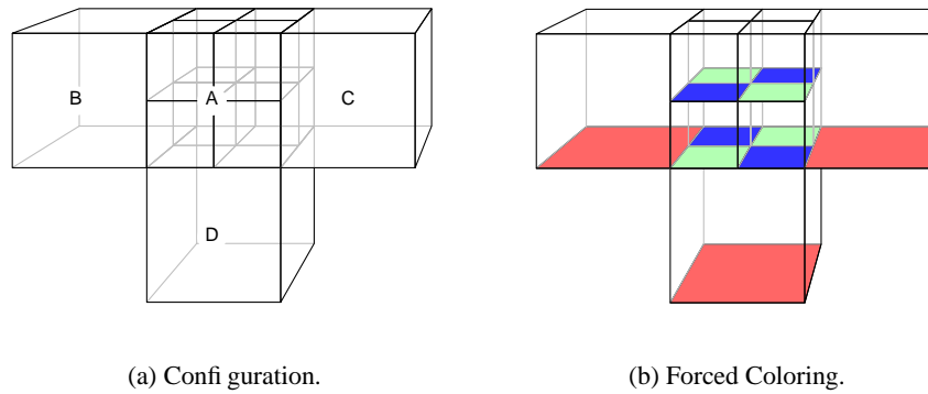
Fig. 3. Illustration for Lemma 3.
